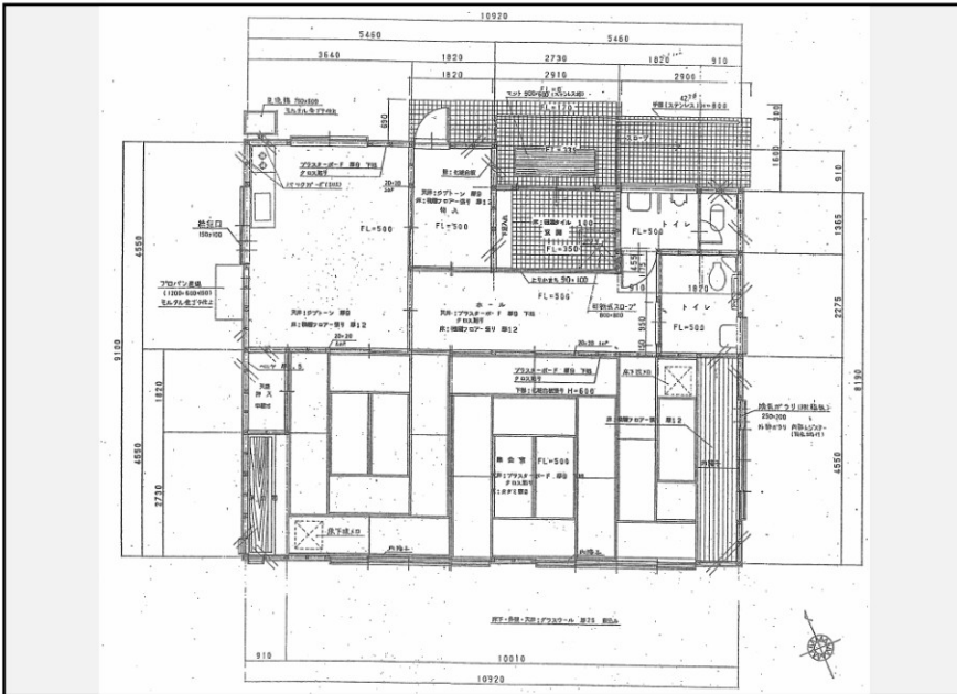
平面図
