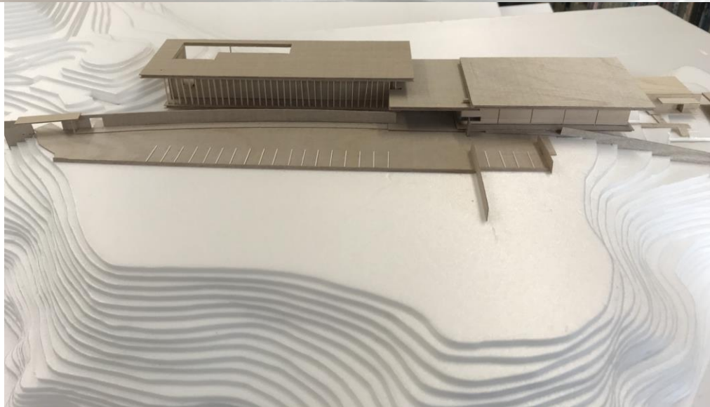
MATER ZONING LAYOUT / 全体配置計画
